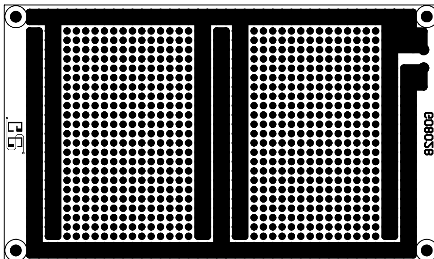
G08028 - Placa Perfurada de 118mmX70MM
